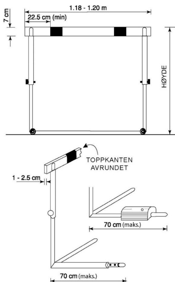
Figur TR 22 – eksempel på hekk
