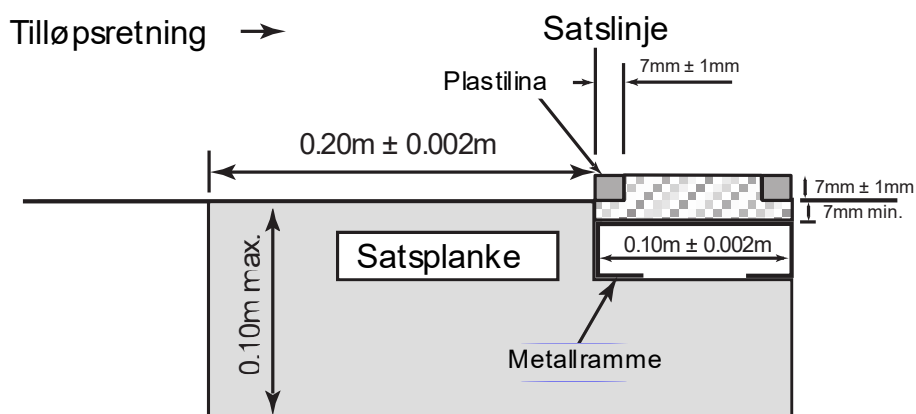
Figur (a2) TR 29 – satsplanke med markeringsbrett med plastelina
