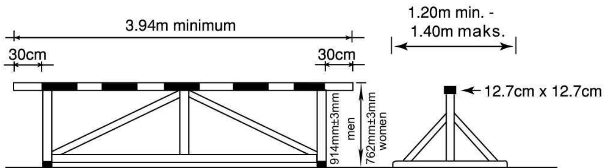
Figur (a) TR 23 – eksempel på et hinder
