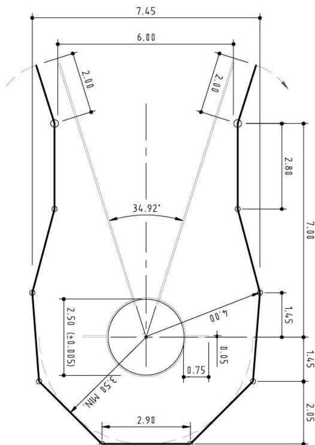
Figur (b) TR 37 – Bur for slegge- og diskoskast med konsentriske ringer (konfigurasjon for diskoskast med dimensjoner til nettet)
