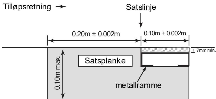
Figur (a1) TR 29 – satsplanke med markeringsbrett
