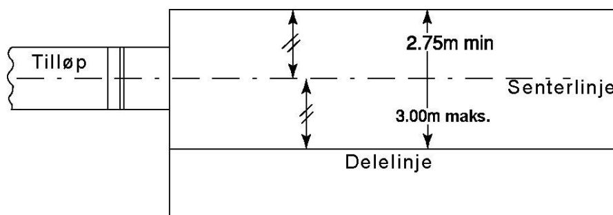
Figur (b) TR 29 – Sentrert landingsområde for lengdehopp og tresteghopp
