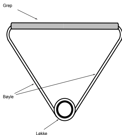
Figur (b) TR 36 – sleggehåndtak
