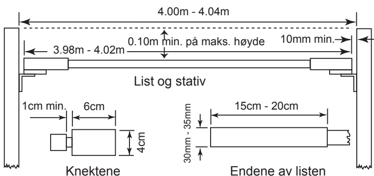
Figur TR 27 – høydestativ og list
