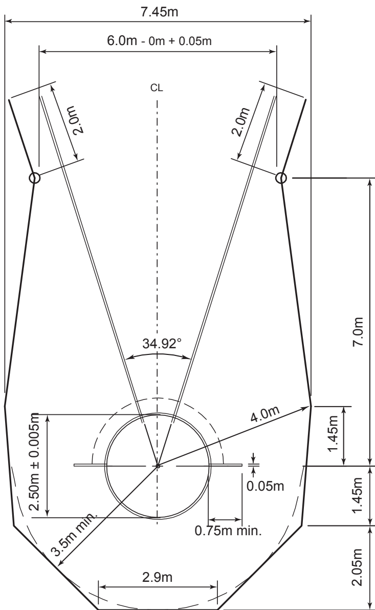
Figur (b) TR 37 - Bur for slegge- og diskoskast med konsentriske ringe (konfigurasjon for diskoskast med dimensjoner til nettet)
