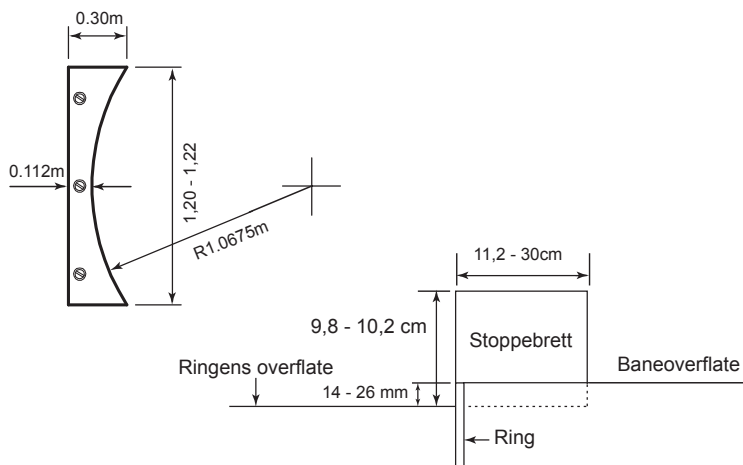
Figur TR 33 – stoppbrett for kulestøt (sett ovenfra og fra siden)
