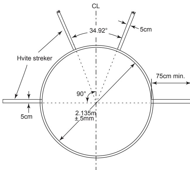
Figur (c) TR 32 - sleggering
