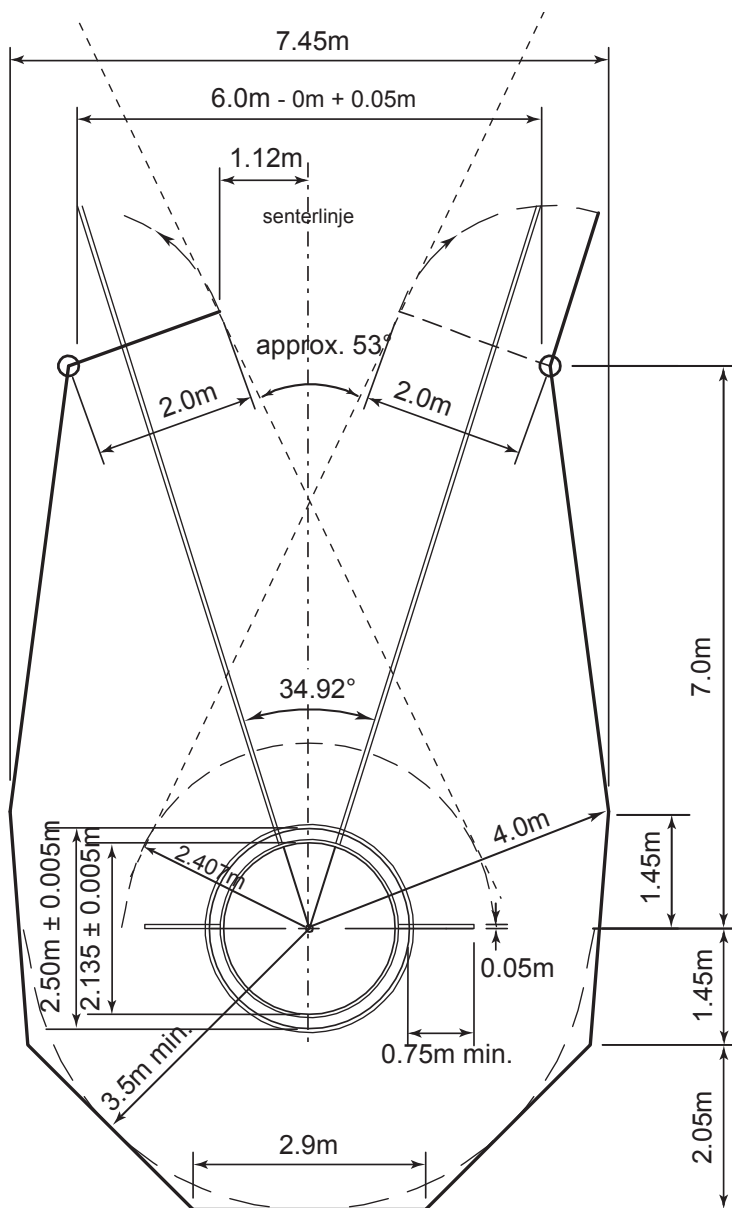
Figur (a) TR 37 – Bur for slegge og diskos med konsentriske ringe (konfigurasjon for høyrehendte sleggekastere med dimensjoner til nettet)
