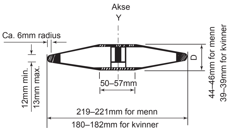
Figur TR 34 - diskos
