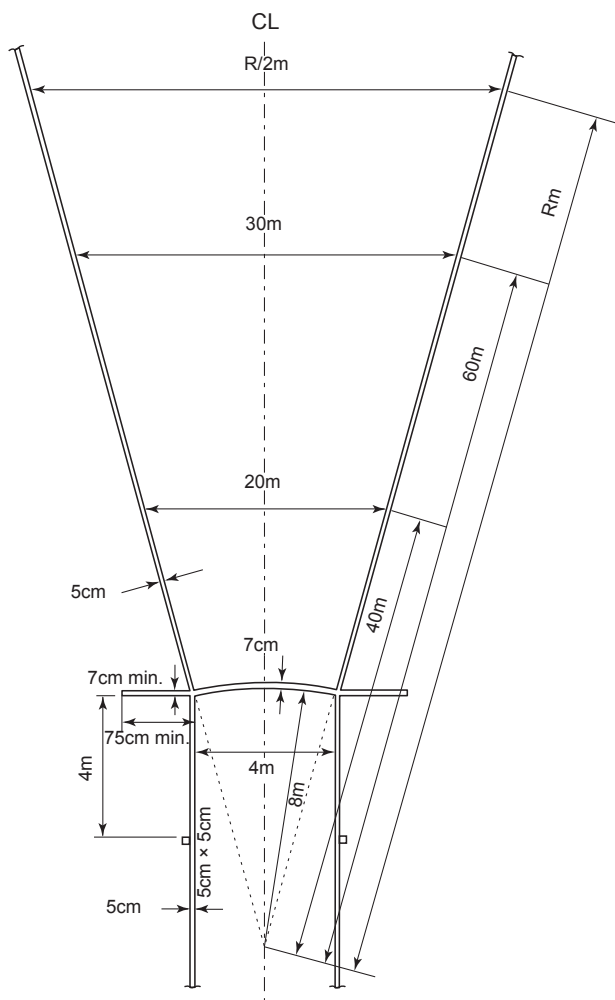
Figur (e) TR 32 - spydtillop og kastsektor
