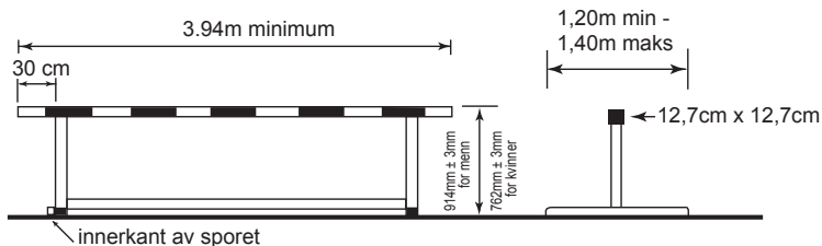
Figur (a) TR 23 – eksempel på et hinder
