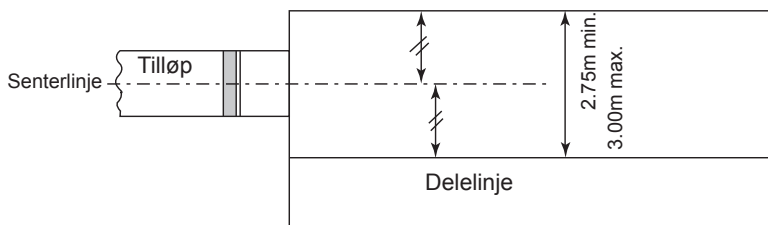
Figur (b) TR 29 – Sentrert landingsområde for lengdehopp og tresteghopp
