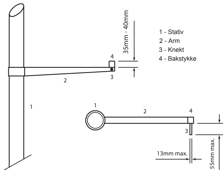
Figur (b) TR 28 – knektene på stavstativet (sett fra matten og ovenfra)
