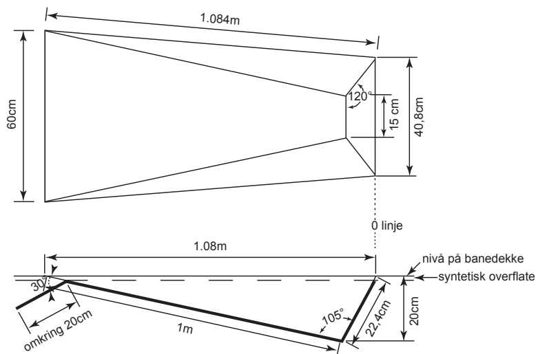
Figur TR 28 – stavkasse (sett ovenfra og fra siden)
