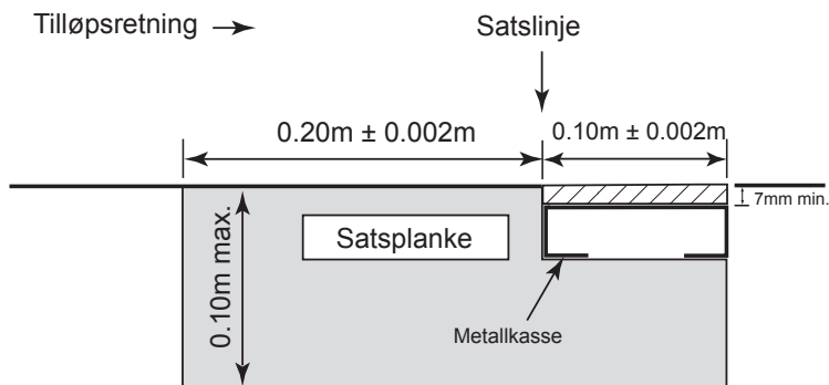
Figur (a1) TR 29 – satsplanke med markeringsbrett
